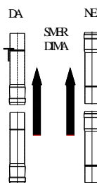
Slika 7. Način montaže dimnih cevi
